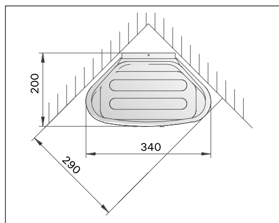
Рисунок 4. Размеры каменки
